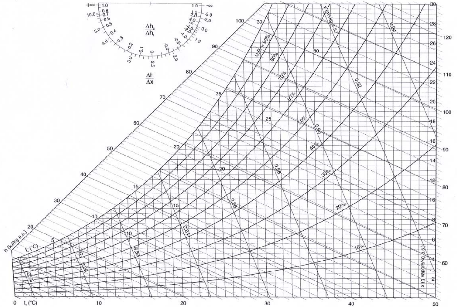
DIAGRAMMA PSICROMETRICO (P = 101,325 kPa)
